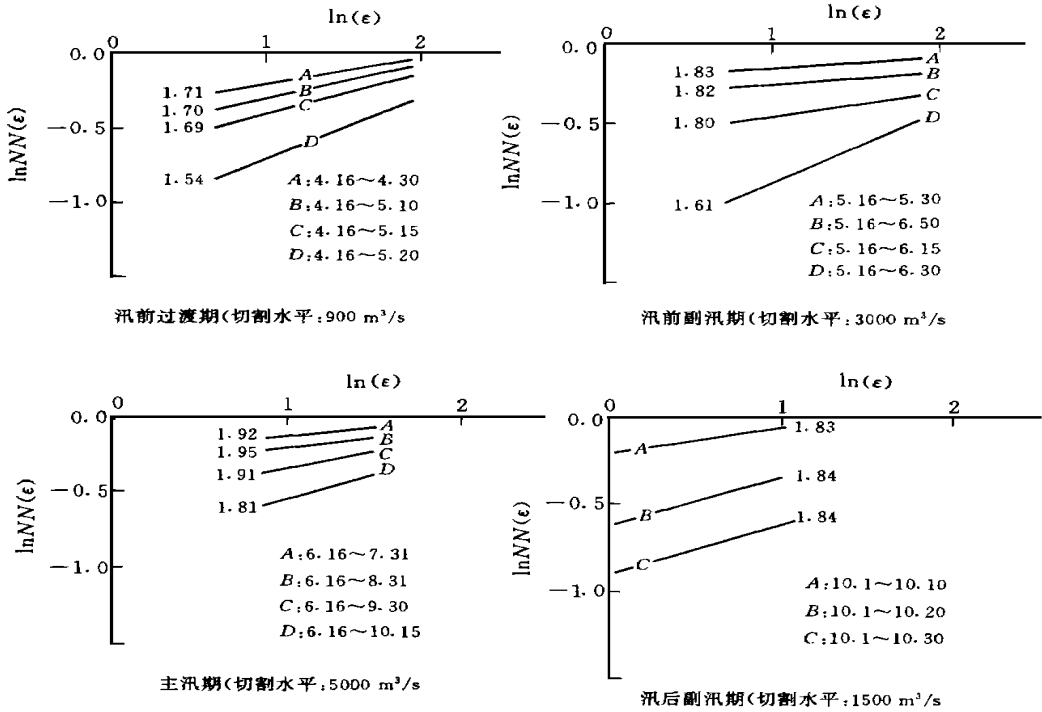
图1 列出在一定切割水平下, 各期 \ln N N(\epsilon) \sim \ln(\epsilon) 关系曲线变化情况。
